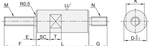
带扳手槽型 OAB51/52/53/56
