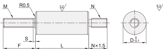
标准型 OAB21/22/23/26
