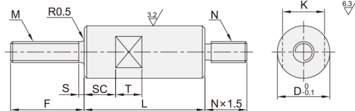
带扳手槽型 OAB31/32/33/36
