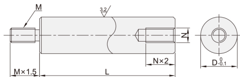
螺纹指定型 OAF21/22/23/26
