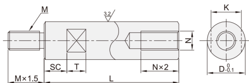
螺纹指定带扳手槽型 OAF31/32/33/36
