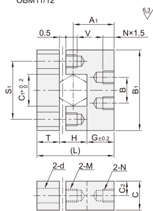
侧面螺纹型 OBM11/12
