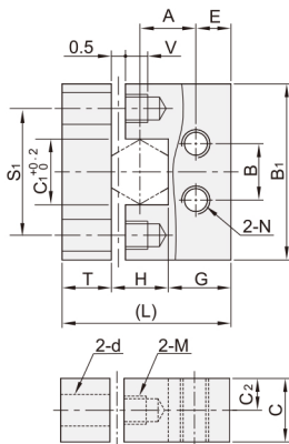
上端螺纹型 OBM01/02
