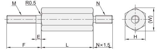
两端外螺纹型 · 一端外螺纹长度指定型 OBG11/12/13/16
