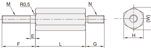
两端外螺纹型 · 两端外螺纹长度指定型 OBG21/22/23/26
