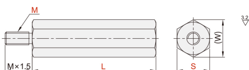
一端外螺纹型 OBB11/12/13/16
