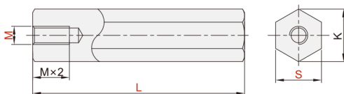
一端内螺纹型 OBB01/02/03/06
