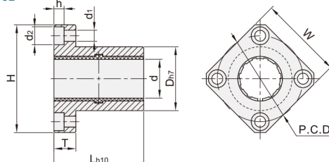
方法兰型 EPS32
