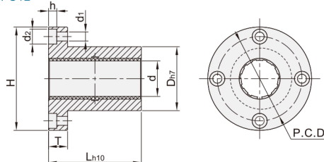
圆法兰型 EPS12
