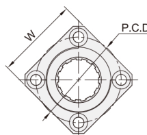
方法兰型 EPS22
