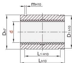
封闭型 EPS11
