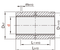
开口型 EPS31
