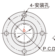
圆法兰型 ELW02MX
