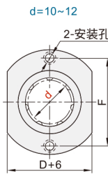
对边法兰型 ELW32MX
