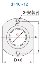
对边法兰型 ELU32MX
