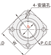
方法兰型 ELU22MX
