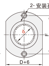
对边法兰型 ELQ32MX/33MX
