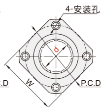
方法兰型 ELQ22MX/23MX
