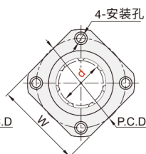
方法兰型 ELP22MX/23MX
