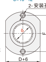
对边法兰型 ELP32MX/33MX
