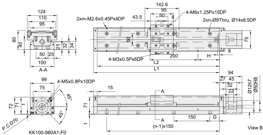
■ 含护盖尺寸图
