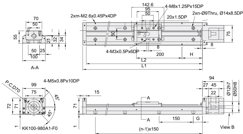
■ 不含护盖尺寸图
