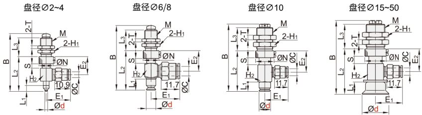
弹簧式侧面真空端口 DSK24/DSK25/DSK26
