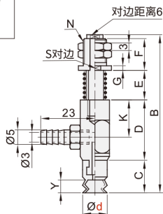
盘径 \varnothing 6/8
