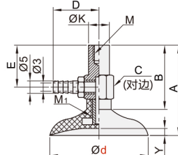
盘径 \varnothing 120-150
