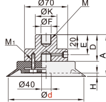
盘径 \varnothing 120-150
