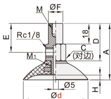
盘径 \varnothing 60-95
