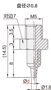
组件 DSR01/02/03/04
