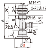
弹簧式侧面真空端口 DSL65/DSL66
