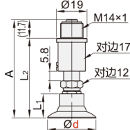
弹簧式直接安装型 DSL67/DSL68
