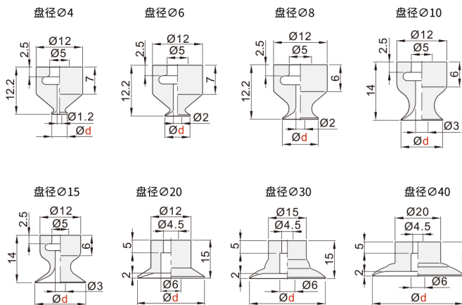
弹簧式侧面真空端口 DSL65/DSL66
