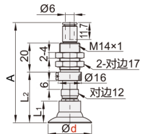
弹簧式直接安装型 DSL67/DSL68
