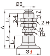
固定式顶部真空端口 DSL61/DSL62
