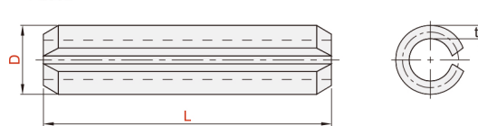
直杆型 PLJ02
