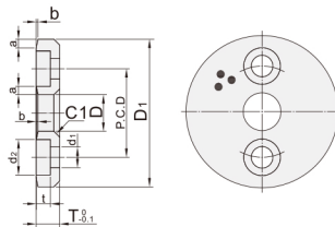
FSG02 沉孔型(内六角薄圆柱头螺钉用)
