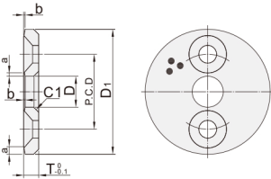
FSG01 锥孔型(内六角沉头螺钉用)
