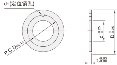
FSH01 止推垫片
