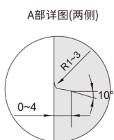
FCE01 标准型同径F7外径m6型
