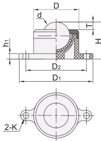
窄耳型 LFH11-25
