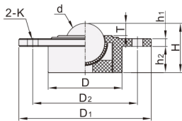
标准型 LFH01
