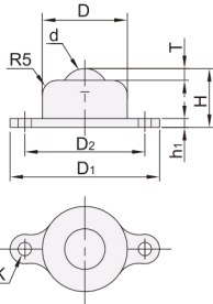
窄耳型 LFH11-16
