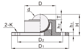
嵌入型 LFH31
