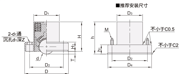
带弹簧向下使用型 LFE72
