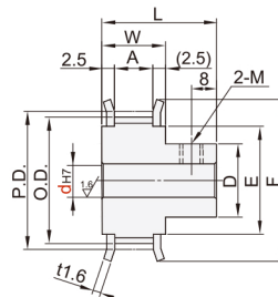
带轮形状: LB形
