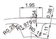
S3M型 (齿距: 3.0)
