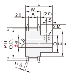
带轮形状: B形
