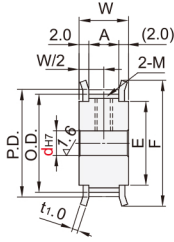
带轮形状: A形
