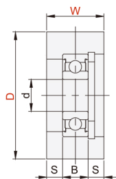
无法兰 单轴承
