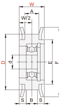
带法兰 单轴承
