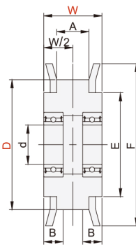
带法兰 双轴承
