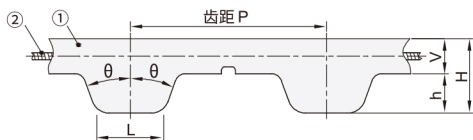
FCX01 标准型 皮带类型: XL/L/H/T5/T10
