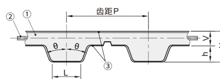
FCX04 两面贴布型
