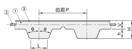
FCX04 两面贴布型
