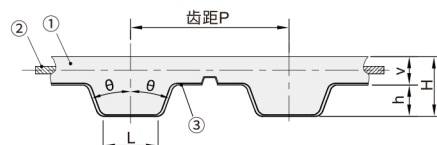
FCX02 齿面贴布型
