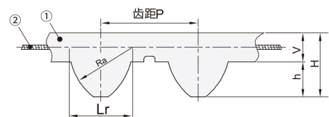
FCX01 标准型 皮带类型: S5M/S8M
