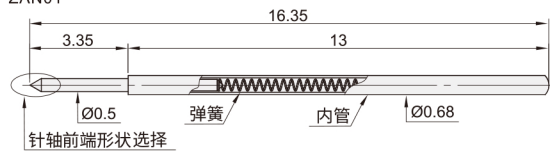
探针 ZAN01
