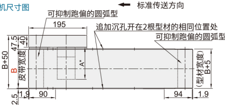
■ 整机尺寸图
