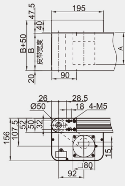
■ 调速\定速\变频电机尺寸(参考值)
