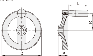
D=140~200
