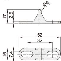
公扣
