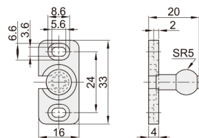
公扣
