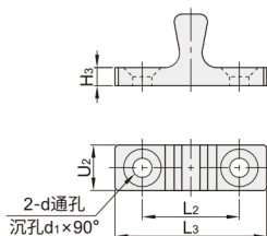
公扣
