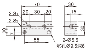
BBC01 30×30
