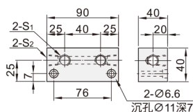
BBC02 40×40
