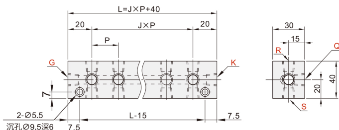
T形端面贯穿 间距固定型 BBR01
