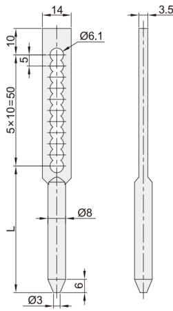
带多孔连杆 XAG41/XAG42
