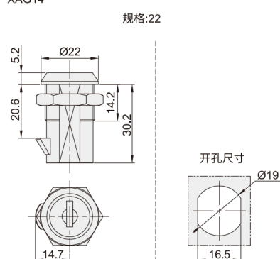
一字形锁芯 XAG14
