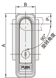
A : 92/110
