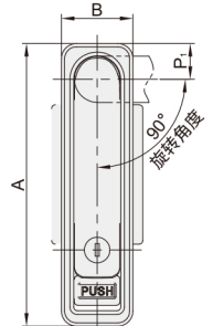
A : 150/170
