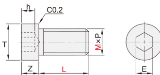
短头小径内六角圆柱头螺钉 YWP13/14
