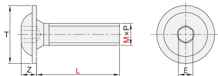
内六角平头带垫螺钉 YWD06/07
