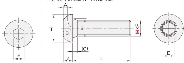
内六角平圆头螺钉 YWG01/02
