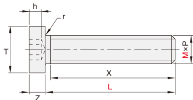
薄圆柱头型 YWV01/02
