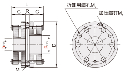
CDK01 单膜片
