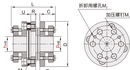
CDK21 双膜片
