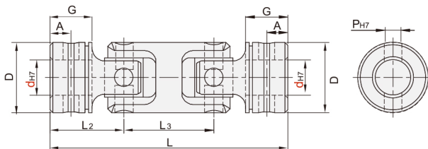
销孔型双节 CXJ21/CXJ72
