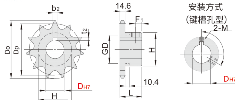
链轮
