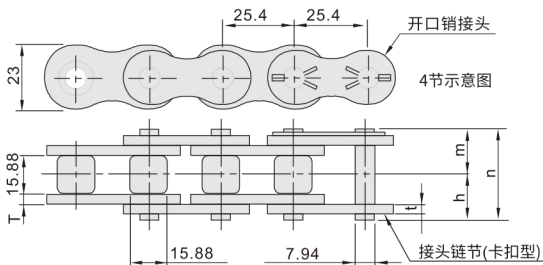
链条
