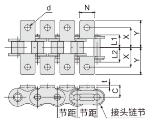
KHZ21□□B (每2节带附件)
