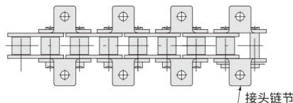
KHZ21□□B (每2节带附件)
