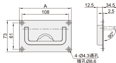
开孔尺寸
