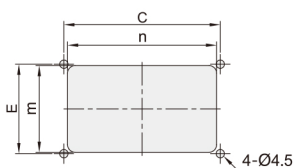
开孔尺寸
