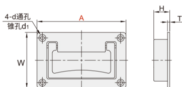
开孔尺寸
