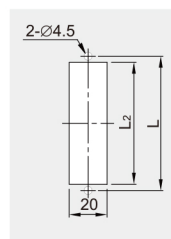
面板安装孔尺寸
