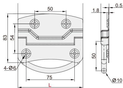
面板安装孔尺寸
