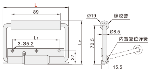
自动复位型 VFW03 VFW05
