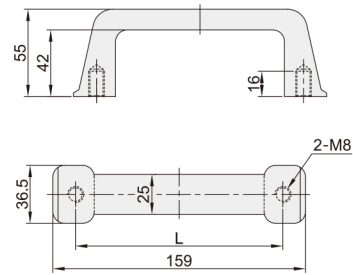
开孔尺寸
