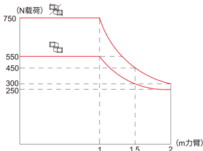
5575系列悬臂组合承重图
