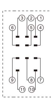
接线图
