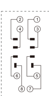
接线图
