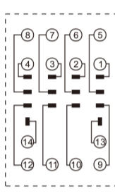
接线图
