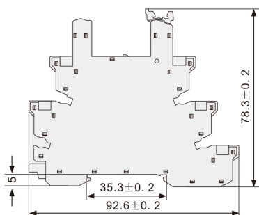
外形及安装尺寸 DUA31
