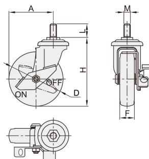
五金边刹 WKF42
